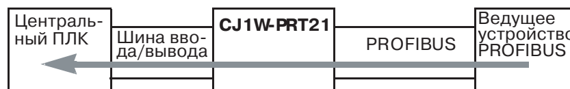
Рисунок 2 Направление передачи выходных данных ведомого устройства
