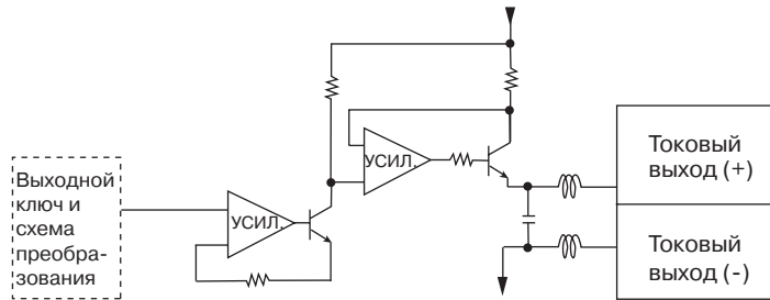
Схема выхода тока
