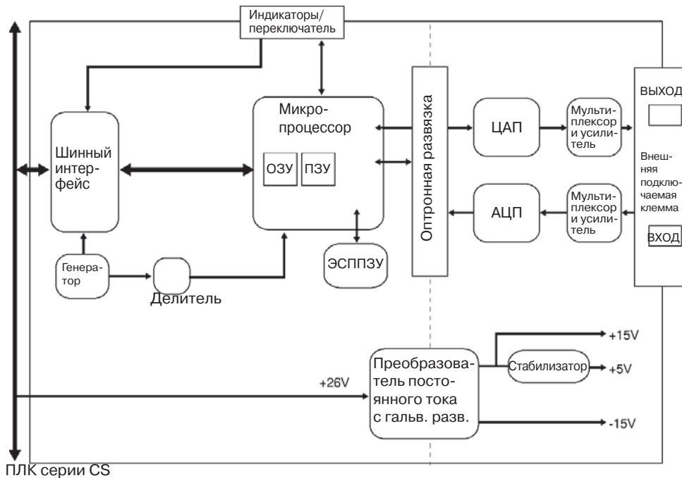
Функциональная схема внутренних цепей
