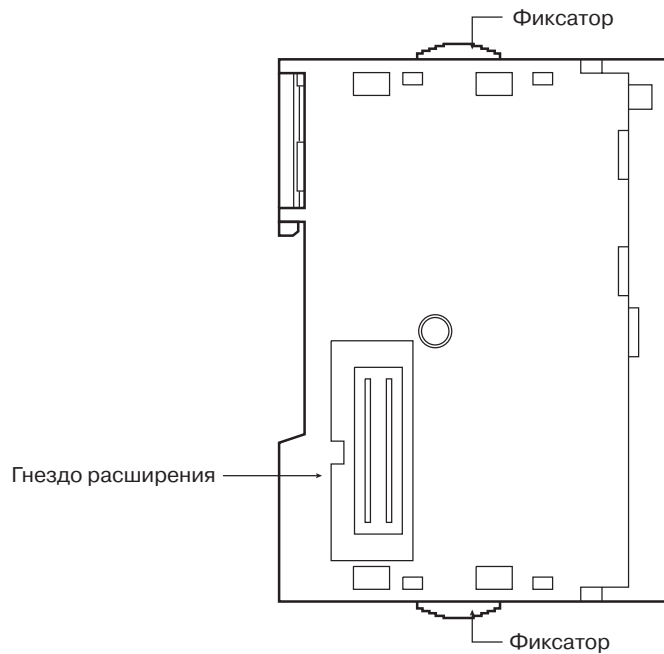
Вид сбоку
