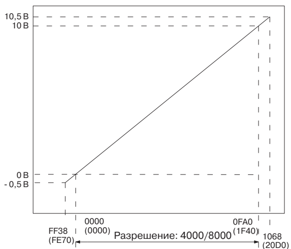
Выходной аналоговый сигнал
