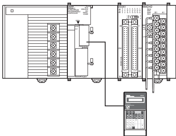
Консоль программирования
