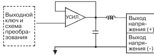
Схема выхода напряжения для CS1W-DA08V/DA041
