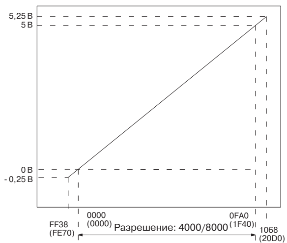
Выходной аналоговый сигнал
