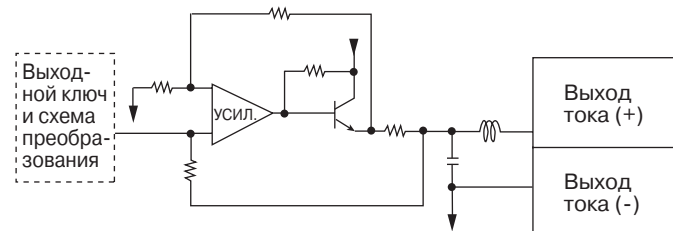
Схема выхода тока для CS1W-DA08C/DA041
