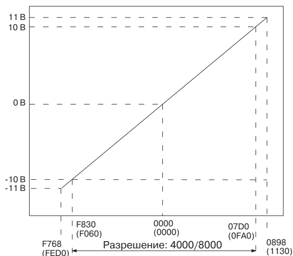
Выходной аналоговый сигнал
