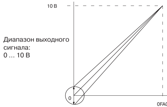
Диапазон регулировки смещения выхода
