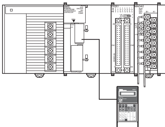
Консоль программирования
