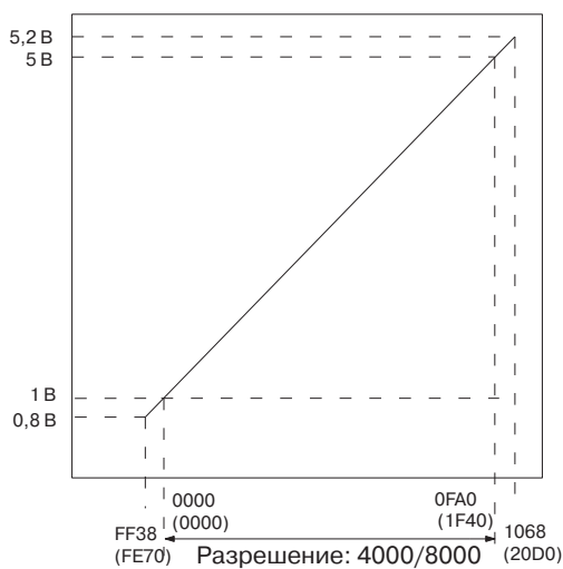
Выходной аналоговый сигнал
