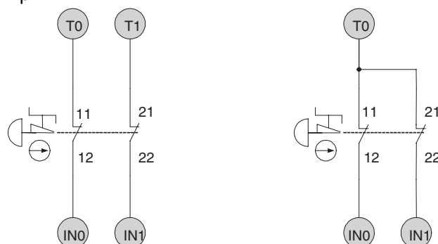
Circuito in cui il rilevamento di un cortocircuito tra i segnali di ingresso è richiesto.
