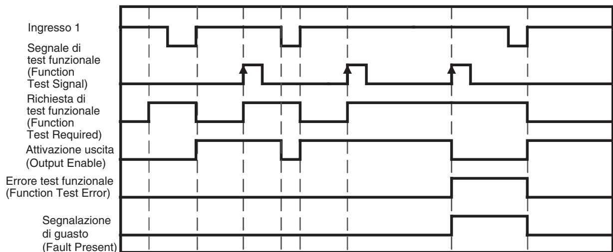
Singolo canale, test funzionale richiesto
