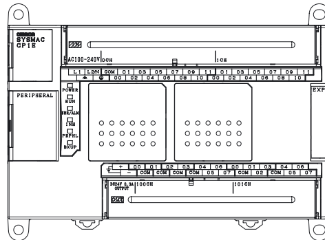
UC de type E CP1E-E40DR-A
