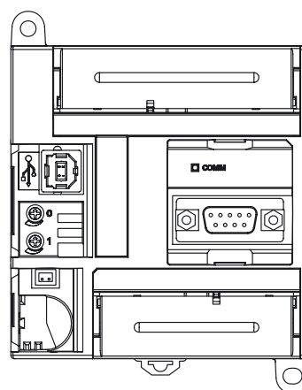
Unidad CPU tipo N CP1E-N20D□-□
