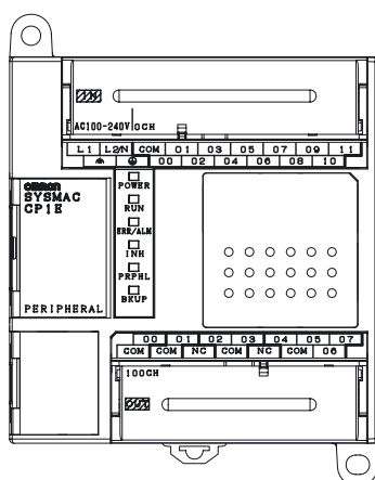
Unidad CPU tipo E CP1E-E20DR-A
