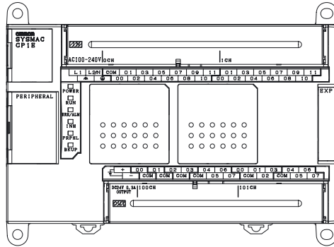
Unidad CPU tipo E CP1E-E40DR-A
