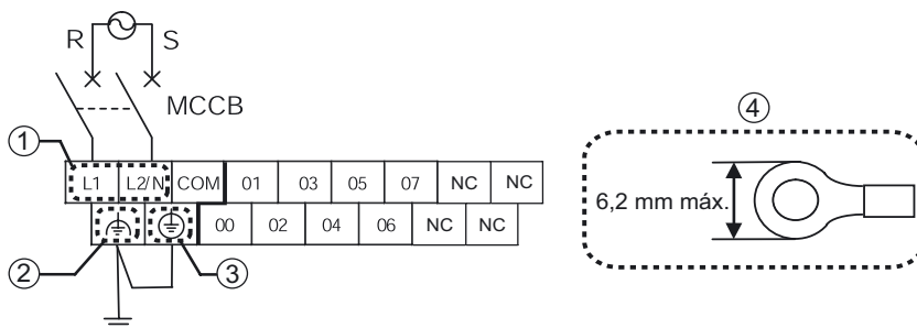
Esquema del bloque de terminales en (A)
