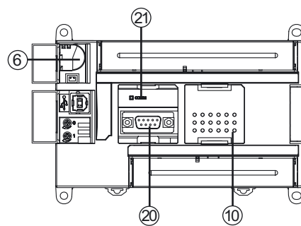
Unidad CPU tipo N CP1E-N40D□-□
