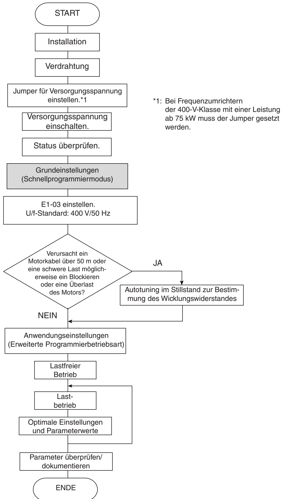
Abb 13 Testbetrieb – Flussdiagramm
