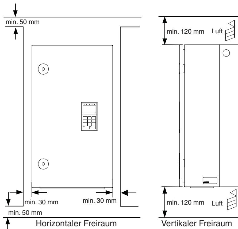
Abb 1 Einbauraum
