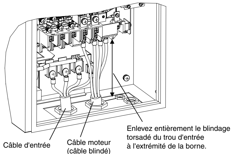
Fig. 8 Blindage des câbles de moteur avec variateur de 22 à 30 kW
