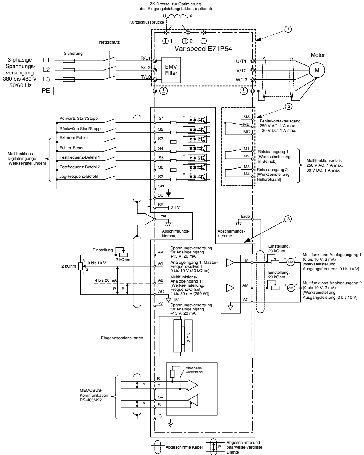
Abb 2 Schaltplan
