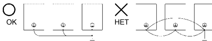
Рис. 7 Выполнение заземления
