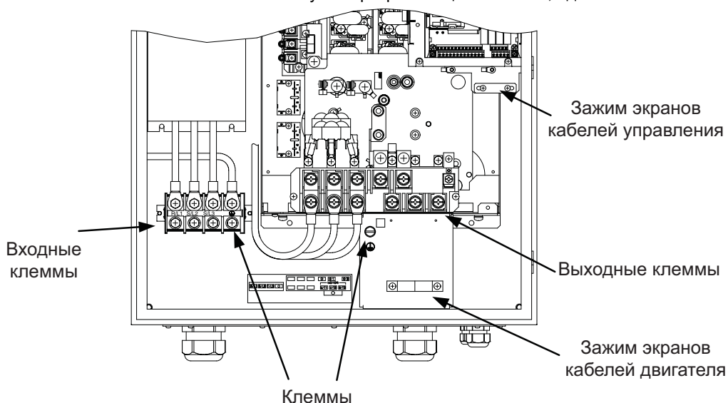
Рис. 3 Расположение клемм у инверторов мощностью от 7,5 до 30 кВт
