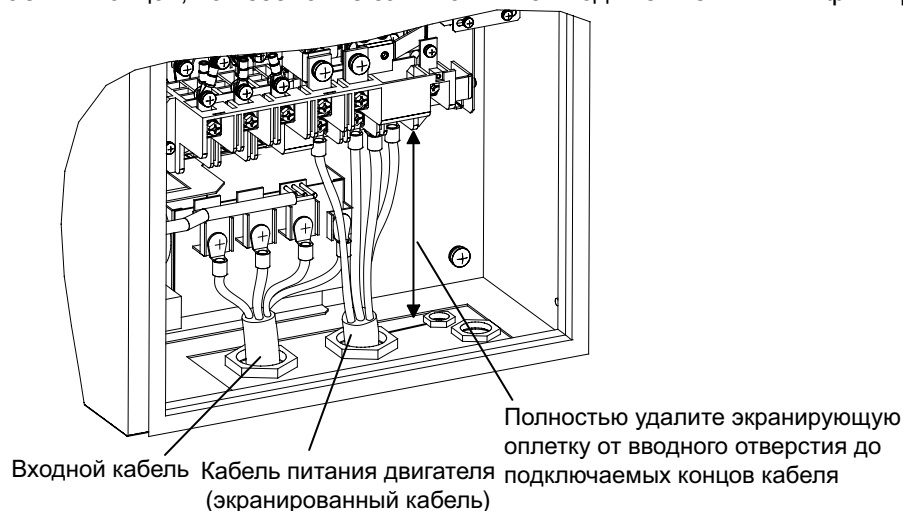
Рис. 8 Экранирование кабеля питания двигателя в инверторах мощностью 22 и 30 кВт
