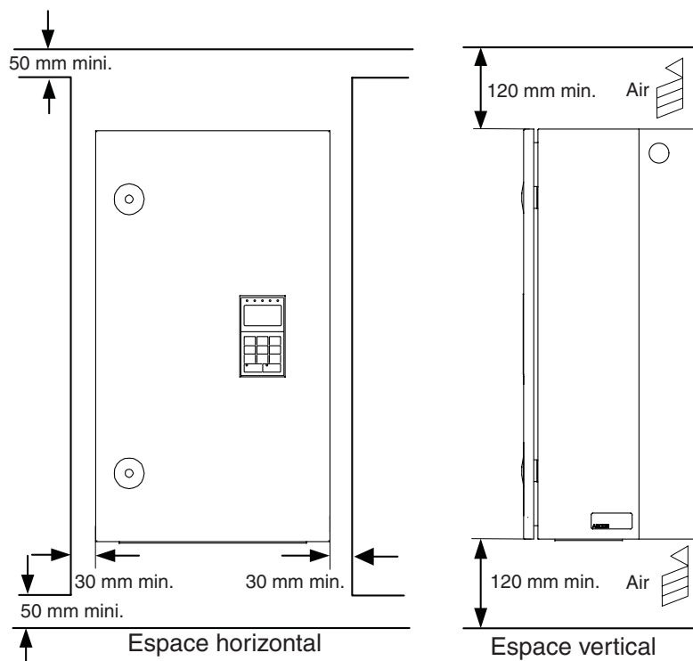
Fig. 1 Espace d'installation
