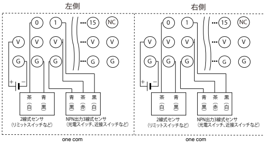
DRT2-ID32SL-1
