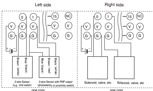
DRT2-MD32SL-1
