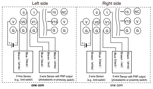
DRT2-OD32SLH
