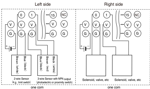
DRT2-MD32SL-1
