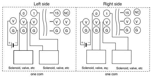
DRT2-OD32SLH-1
