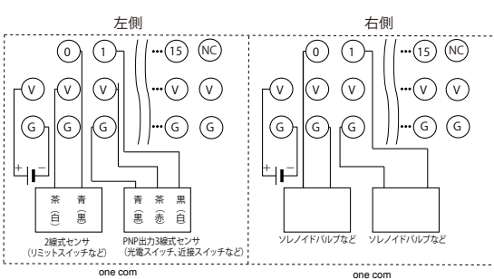
DRT2-MD32SL-1
