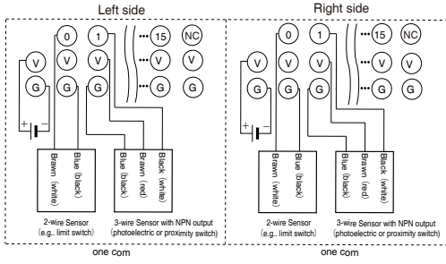
DRT2-ID32SL-1
