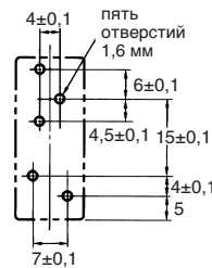
Крепежные отверстия
