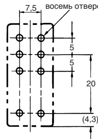
Крепежные отверстия
