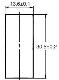
Монтажный вырез
