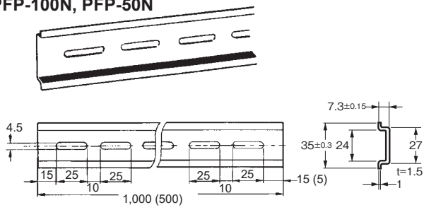
PFP-100N, PFP-50N
