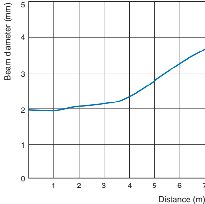
E3C-LR12N
