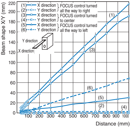
E3C-LD11N + E39-P11
