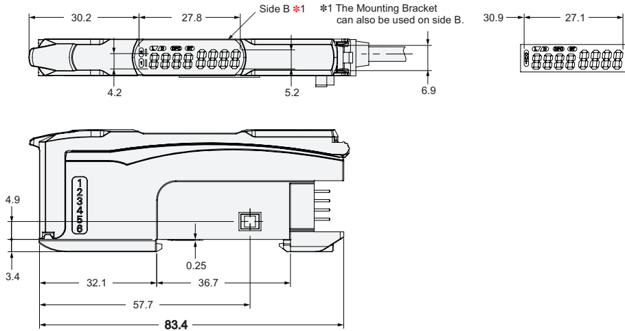
E3C-LDA6N/LDA8N
