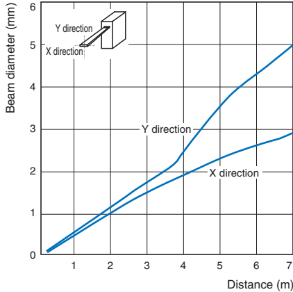
E3C-LR11N
