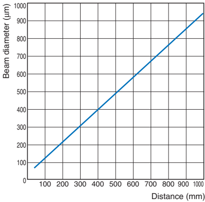
E3C-LD11N
