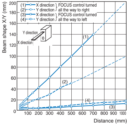
E3C-LD11N + E39-P21
