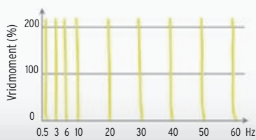
Frekvensomfång kontra vridmomentsvariation Exempel med 7,5 kW fyrpolig motor
